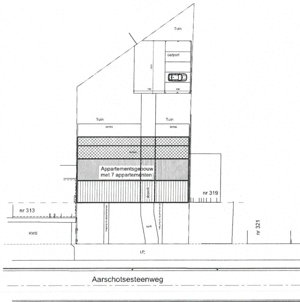
Grondplan carport
