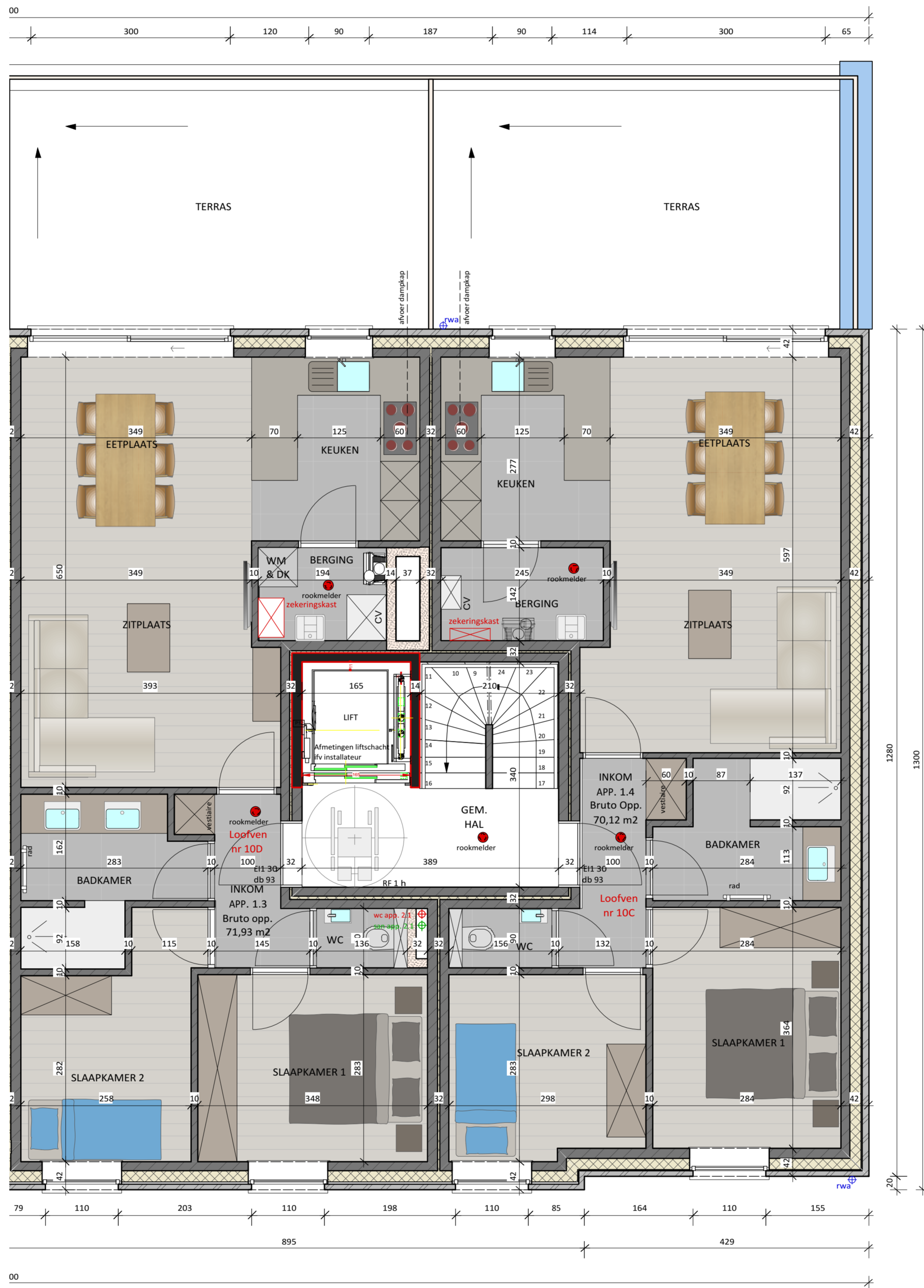
1ste Verdieping Loofven nr 10 SCHAAL 1/50
