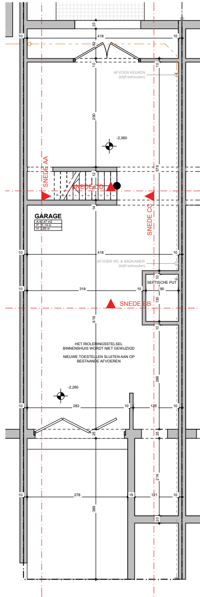
BT KELDER/GARAGE 1:50
