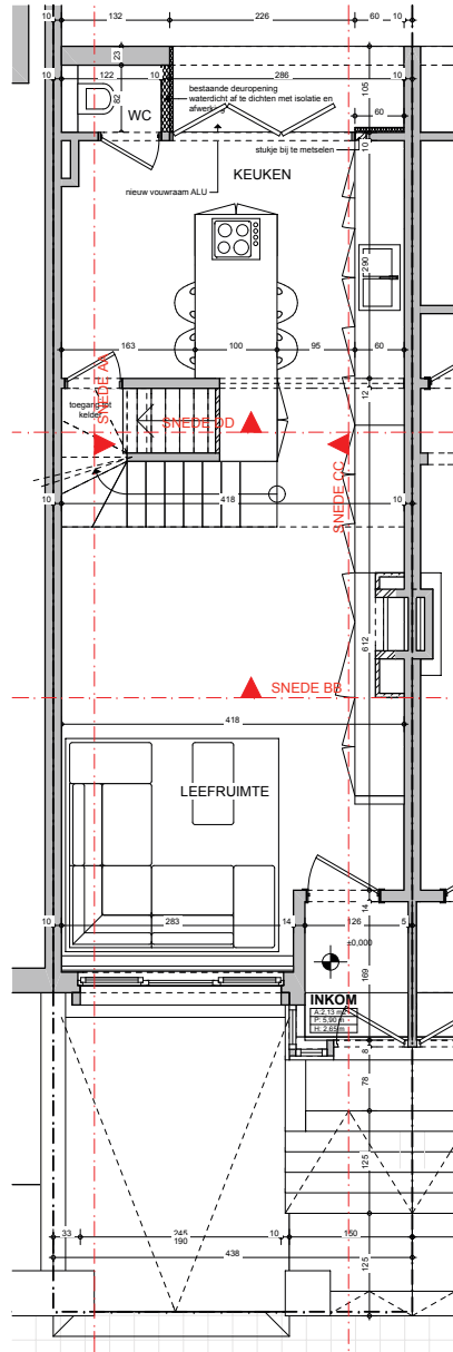
BT GELIJKVLOERS 1:50
