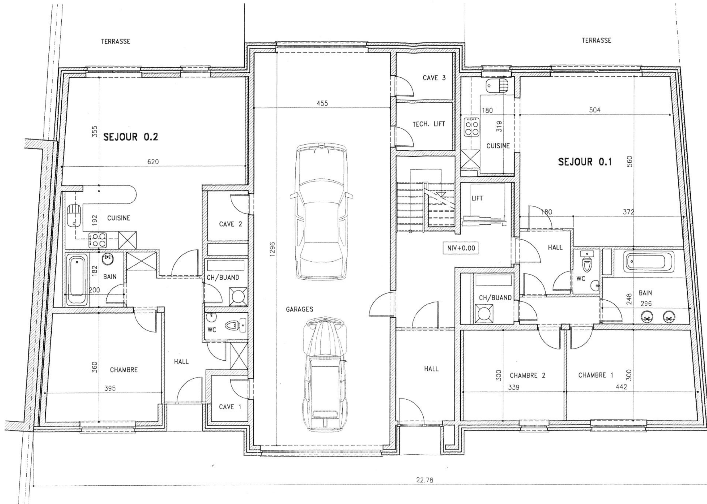
PLAN DU REZ-DE-CHAUSSEE
