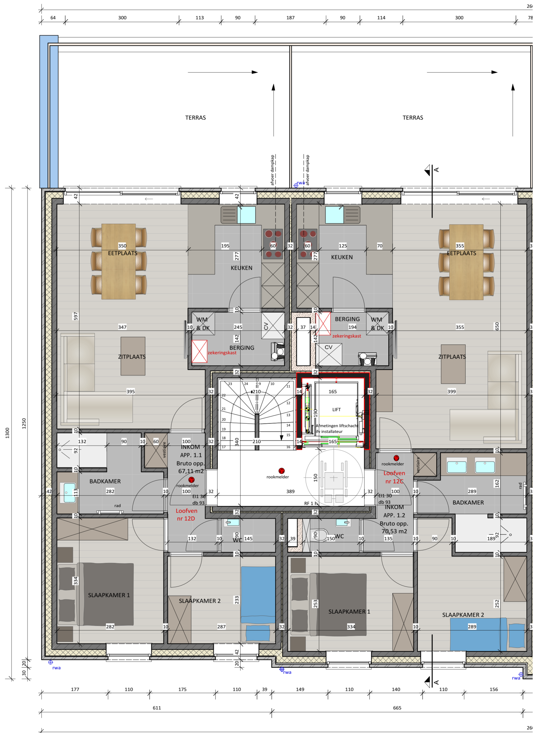
1ste Verdieping Loofven nr 12 SCHAAL 1/50
