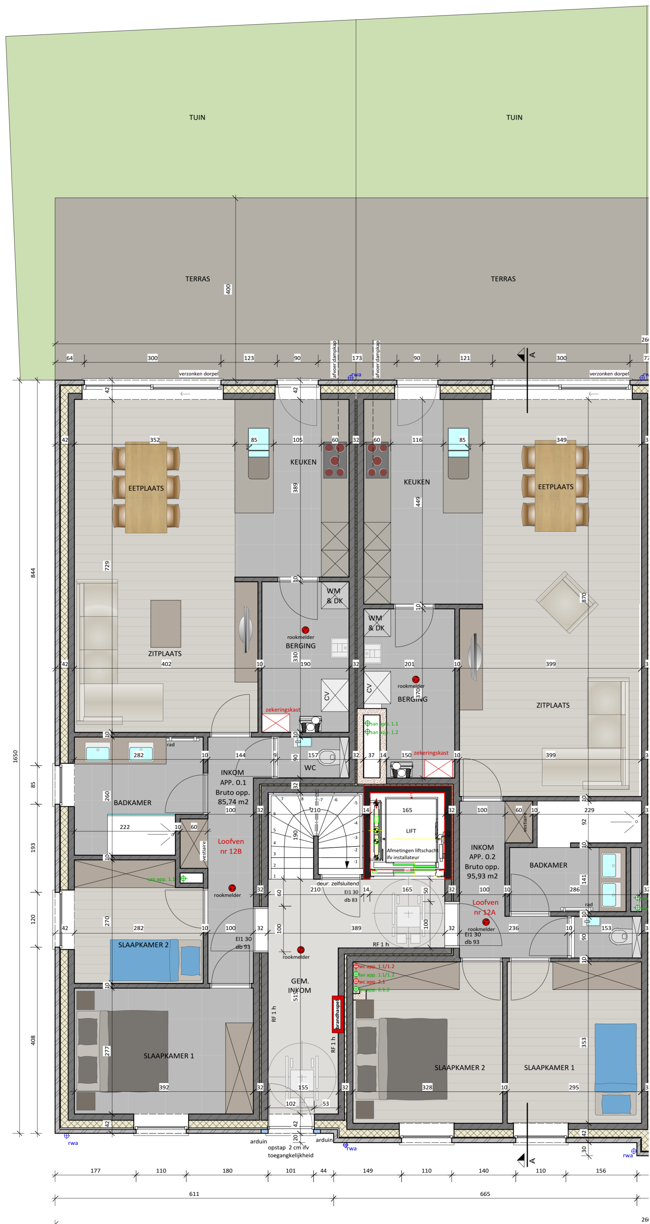
Gelijkvloers Loofven nr 12 SCHAAL 1/50
